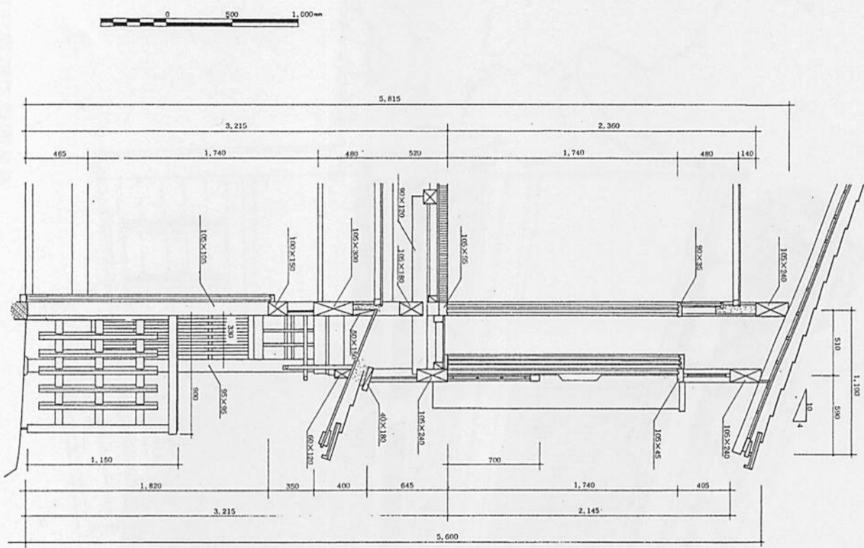
出格子詳細
