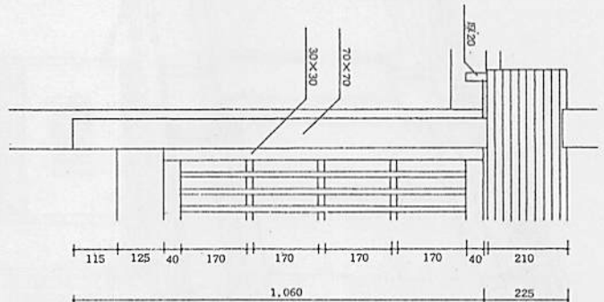
つり格子 詳細
